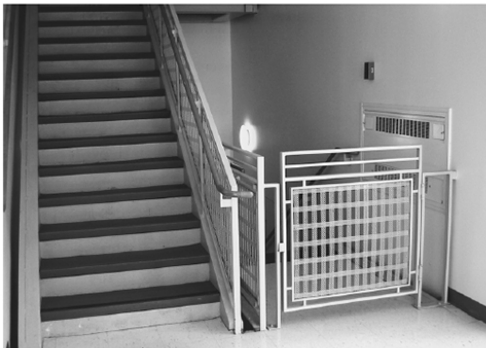
HÌNH 4.7 Chức năng bắt buộc theo cơ chế khóa ngăn ngừa cho cửa thoát hiểm khi có hỏa hoạn. Cánh cửa được đặt tại cầu thang tầng trệt, ngăn không để những người đang chạy thoát thân đi tiếp xuống khu vực tầng hầm, nơi họ có thể bị mắc kẹt.
